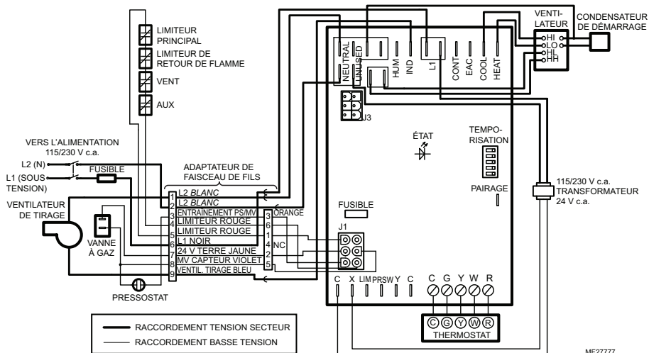
Fig. 3. Schéma de raccordement type du ST9120U,B dans un système ST9101.
