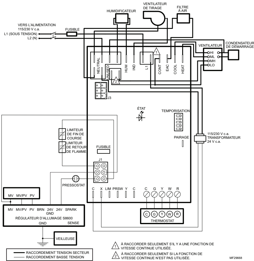
Fig. 1. Schéma de raccordement type du ST9120 à un module pour système d'allumage à veilleuse intermittente S8600.
